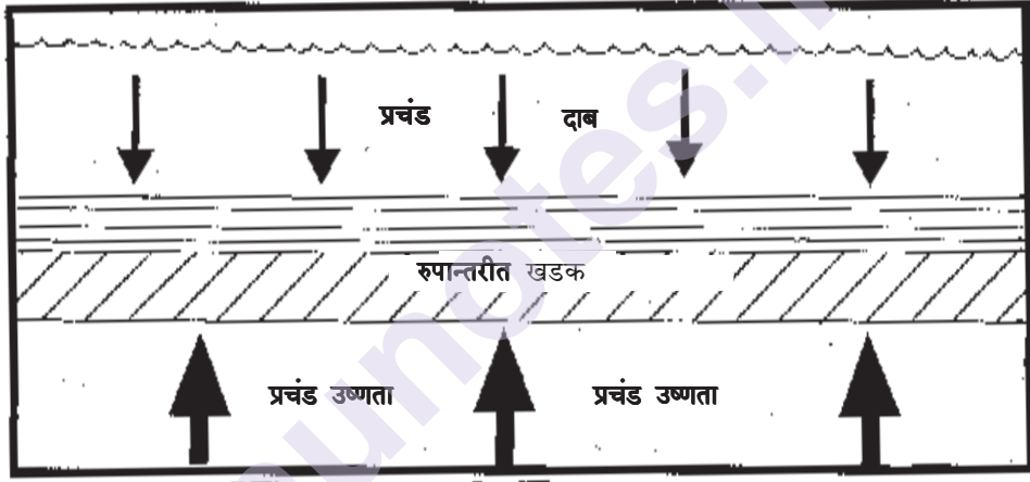
आकृती २.७ : रुपांतरीत खडक
